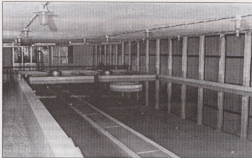
Notranost vodarne na Levstikovi ulici v Il. Bistrici. Čistilno napravo z usedalniki in filtri bi morali razširiti, ker je njena kapaciteta le 72 l/sek, v sušnih obdobjih pa črpa mnogo večje količine.
