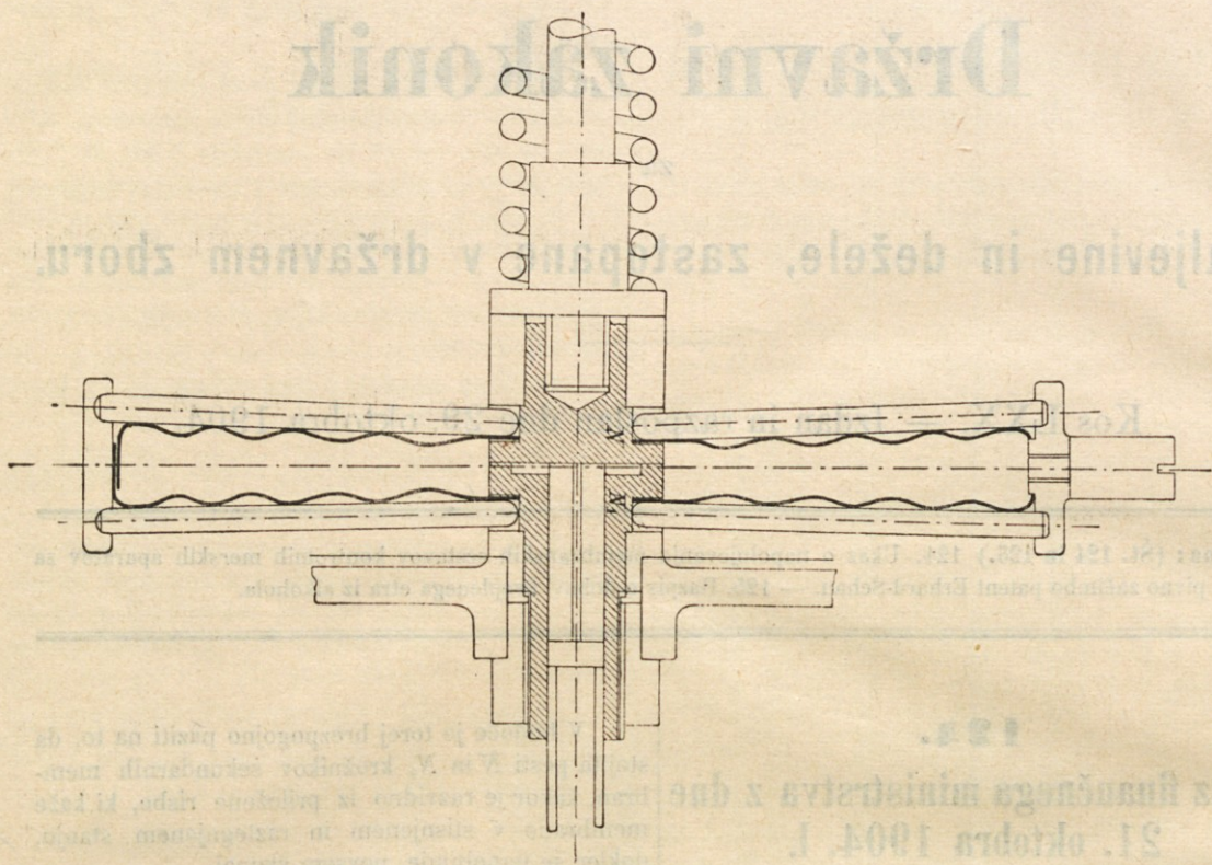
Sekundarna membrana stisnjena, torci v polnilnem stanju.
