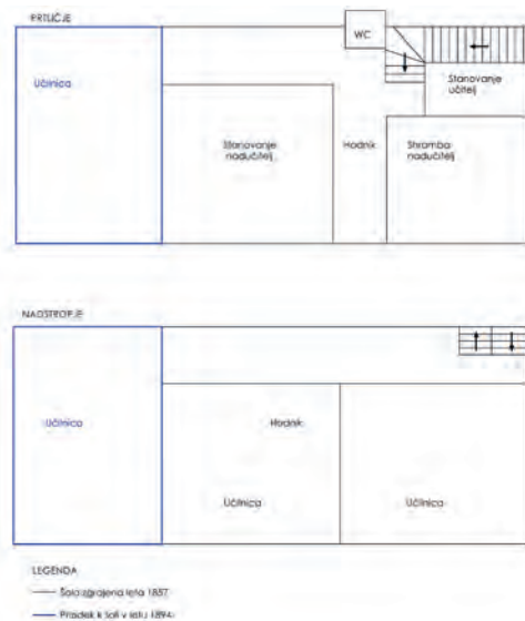
Tloris šolske stavbe po preureditvi prostorov leta 1901. 9
