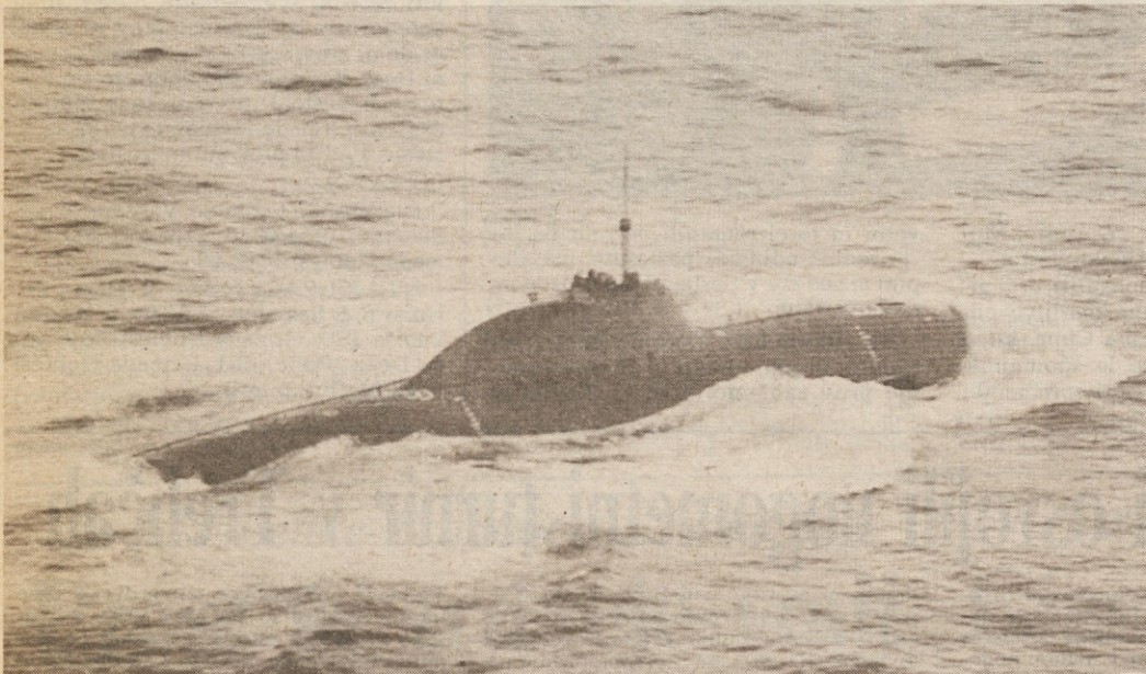
Sovjetska jedrska podmornica razreda alfa, ki ima 2.900 BRT, dva jedrska reaktorja, štiri dizelske motorje in ki je oborožena z jedrskimi raketami SS 15 (Telefoto AP)
