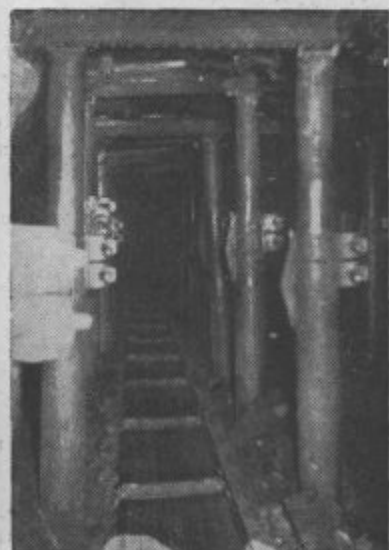
Pogled vzdolž širokega čela podgrajenega v popolnem jeklenem oporju in z dvoverzišnim transporterjem za odvoz odstreljenega premoga
