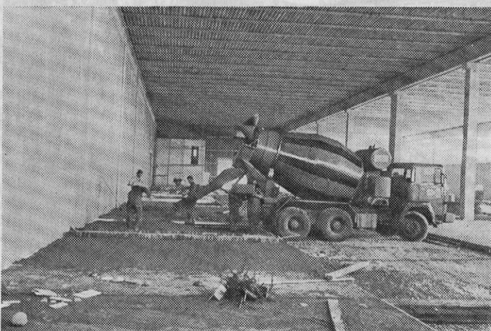
Zaključevanje del v notranjosti
