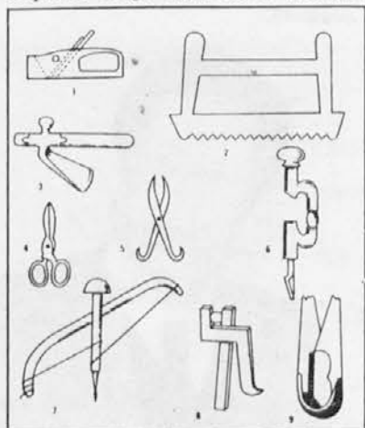
Utensili di epoca romana: 1) pialla (Pompei); 2) sega (Roma); 3) accetta a martello (Gallia); 4) forbici (Ronsen); 5) forbici (Priene); 6) girabecchino (Napoli); 7) trapano (Tebe); 8) fustella (Autun); 9) cesole a lama intercambiabile (Pompei)
