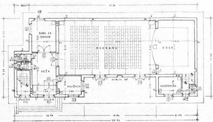
Načrt nove dvorane Mar. doma v Rojanu
