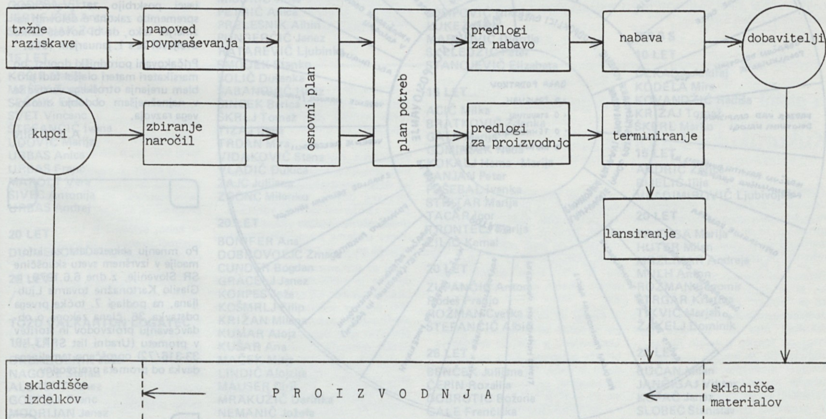
SLIKA 3: Osnovni tokovi informacij pri krmiljenju proizvodnje
