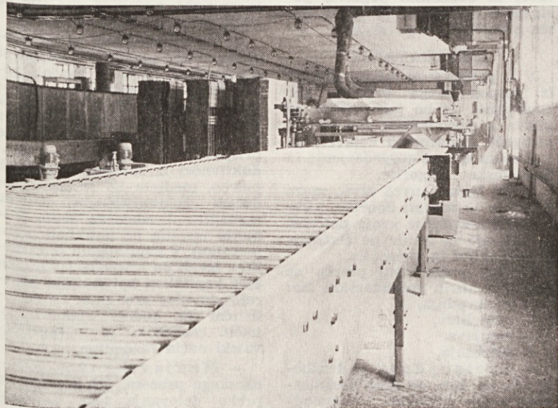
Sušilni kanal v TP Cerknica ob končni montaži
