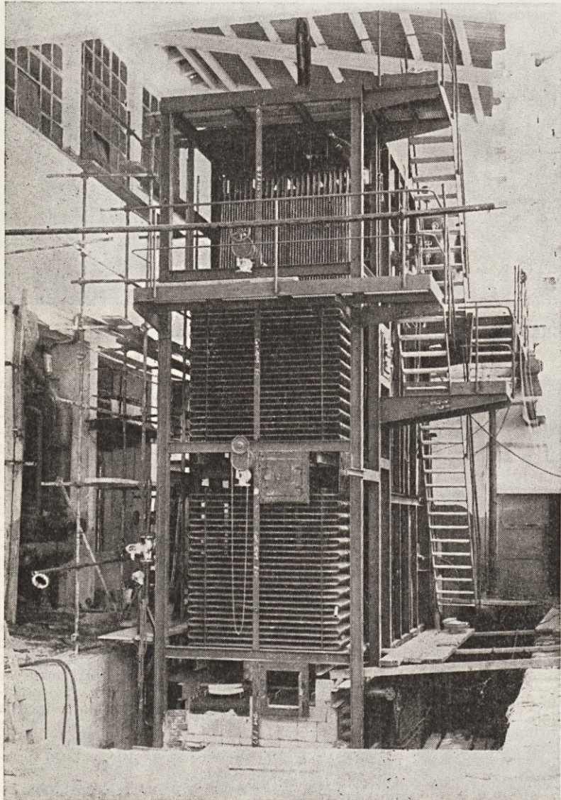
42-atmosferski parni kotel Streicher iz Zah. Nemčije v gradnji
