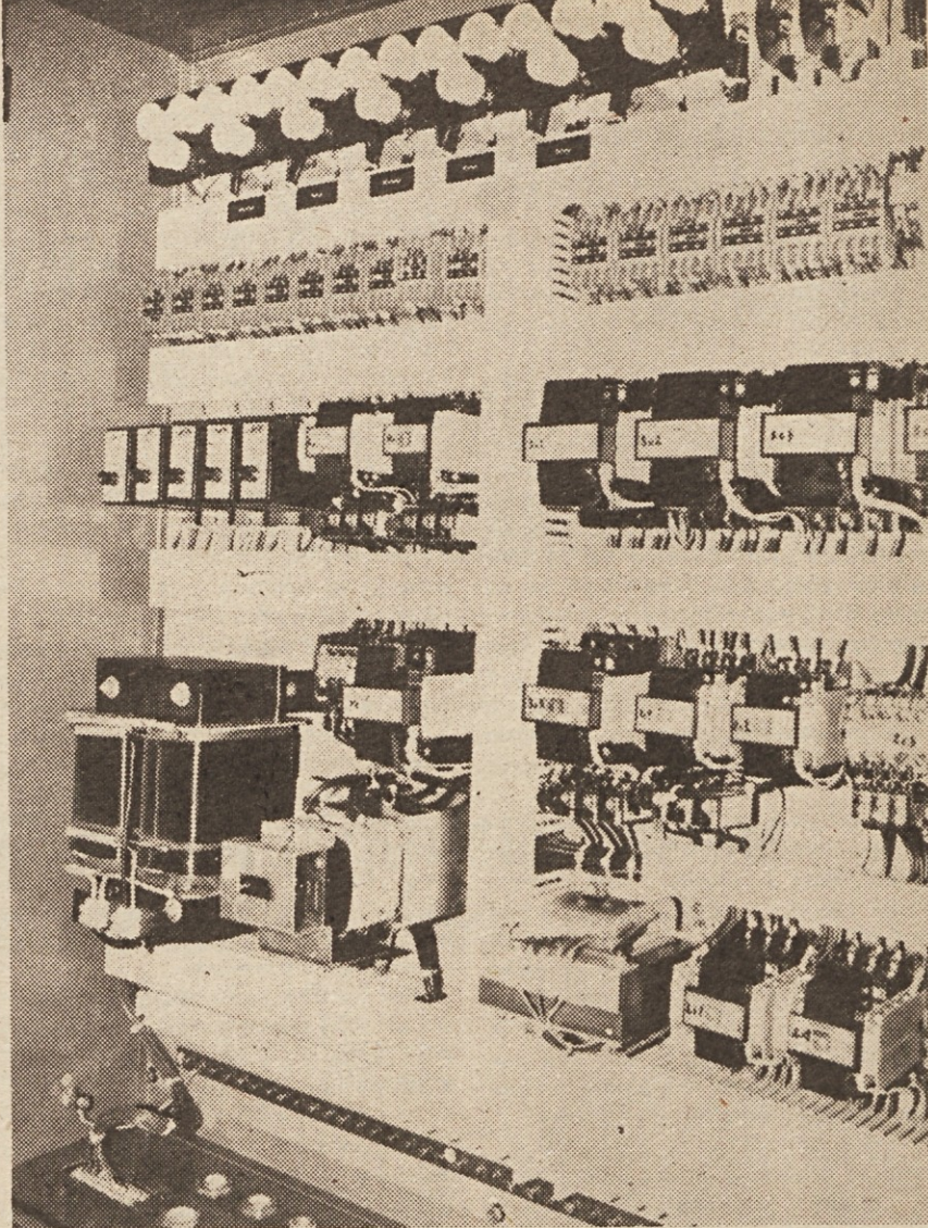
Posnetek kaže kontaktorsko omaro za gradbeni žerjav. To je izdelek Industrije za telekomunikacije, elektroniko in elektromehaniko, TOZD Stikala v Kranju, na katerega so zelo ponosni. Današnja reportažo smo pripravili iz TOZD Stikala in jo objavljamo na 4. in 5. strani.
