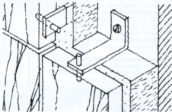
Oblaganje fasade s kamnom "na suho" - tipični primer obešene, prezračevane in toplotno izolirane fasadne strukture. Debelina sidra določa tudi širino fuge.
