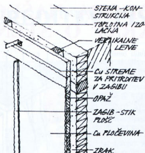
Fasadna obloga iz bakrene pločevine na opažu.
