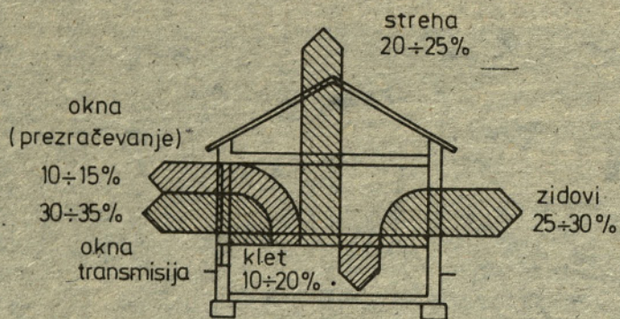
Toplotne izgube enodružinske hiše.
