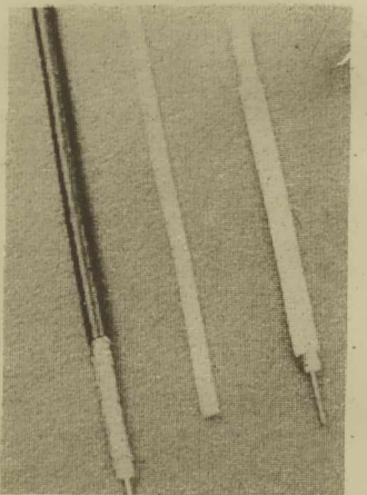
— Črni kabel na levi — koaksialni kabel z votlim dielektrikom — je Pečirerjeva tehnična izboljšava, v sredi je poskusni kabel in desno vzorec francoske firme SIVA.
