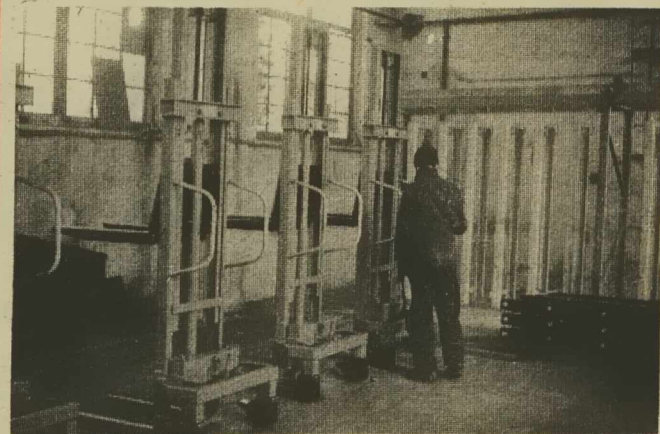
Viličarji iz Lendave so izdelani v glavnem iz domačih surovin in reprodukcij materialov ter domačega znanja. Vsi izdelki, ki jih bodo naredili letos, so že prodani.
