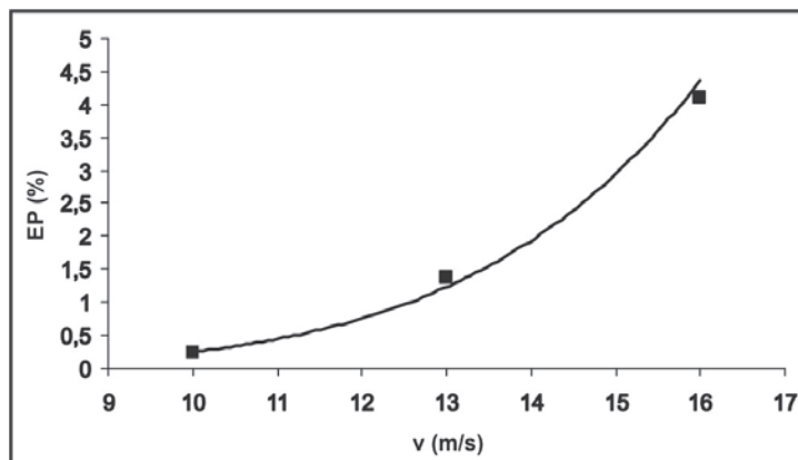
Sl. 11. Erodirana površina ( EP ) kot funkcija hitrosti toka
