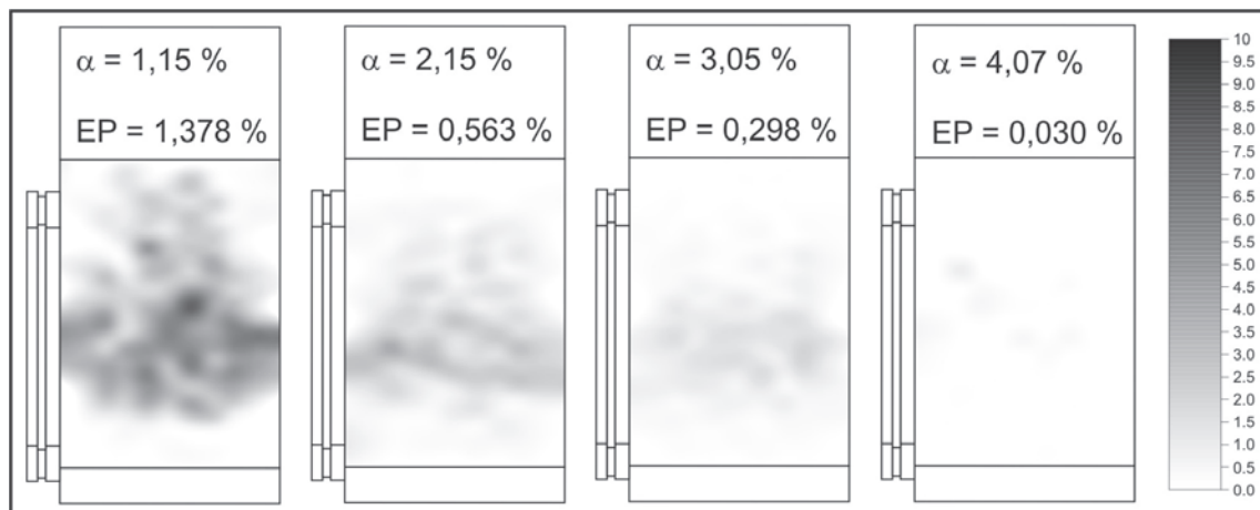
Sl. 8. Porazdelitev velikosti poškodbe za različne deleže plinov v vodi
