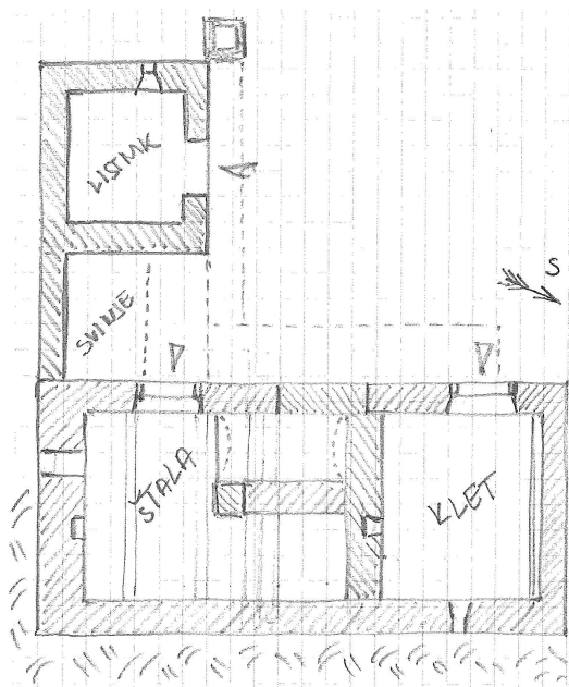
Slika 104: Tloris kleti Matijeve hiše, z različnima šrafurama sta označeni (vsaj) dve fazi zidave. Osnova je velika 11x4,9m.
