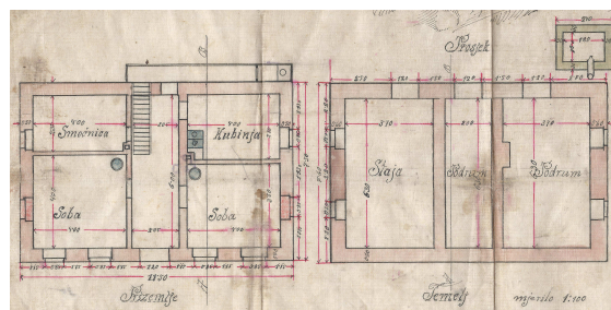
Slika 149: Risbe iz gradbenega načrta Šafarjeve hiše v Gašparcih iz leta 1921. Iz arhiva Šafarjevih.
