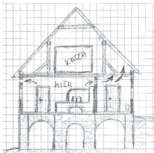
Slika 277: Poskus rekonstrukcije prereza dimnične Pintarjave hiše v Križevi Dragi, iz prve polovice 19. stoletja, po tlorisih.
