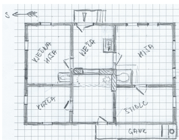
Slika 245: Tloris kleti in rekonstrukcija nadstropja Klukavčave hiše v Črnem Potoku, s črno kuhinjo. Klet je dimenzij približno 11,2x7,6m.
