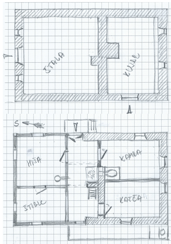
Slika 196: Tloris kleti in poskus rekonstrukcije nadstropja pri Zajskih, v tretji četrtini 19. stoletja. Vprašljiv je levi del z vežo in sobama, saj ni logičen po shemah tedanjega časa. Verjetno je posledica večih družin v eni hiši. Dimenzije kleti so 11,3x6,9 m.
