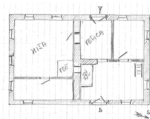
Slika 232: Tloris kleti in rekonstrukcija nadstropja Grgečave hiše iz obdobja črne kuhinje v drugi polovici 19. stoletja, zunanjih dimenzij približno 7,7x12,2 m.
