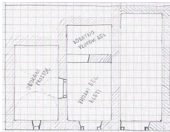
Slika 224: Tloris sedanje kleti Petričkave hiše. Levi del dveh tretjin, ki v osnovi z zunanjimi stenami tvori kvadrat 7,6x7,6m je vsaj iz sredine 19. stoletja, polkrožno obokana klet levo pa celo kako stoletje starejša. Hiša je morala biti prvotno v delu nad sedanjim srednjim vhodom in obokano kletjo, v fazi s črno kuhinjo pa v levem kotu. Stavba je sedaj zunanjih dimenzij približno 10,3x8,3m leva.
