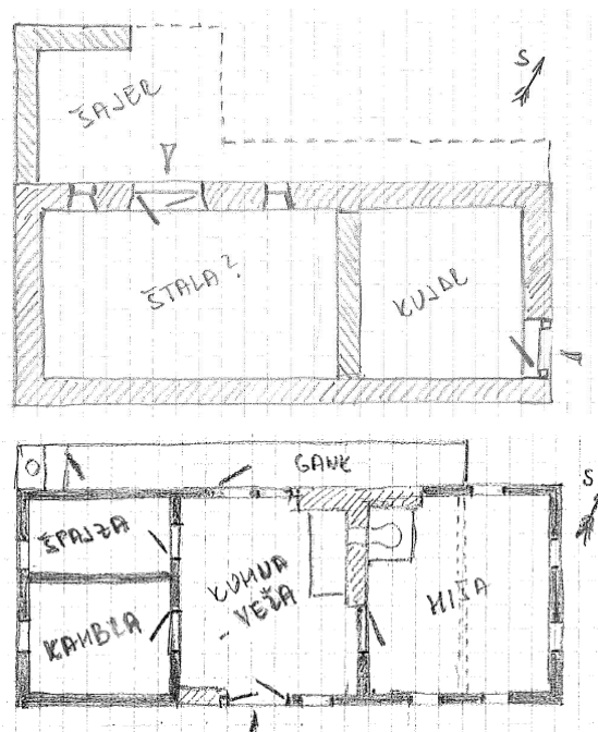
Slika 121: Tloris kleti in poskus rekonstrukcije nadstropja hiše, ko je imela še črno ali celo kuhinjo z nizkim ognjiščem in je bila brez prizidanega ključa, v sredini 19. stoletja. Osnovne dimenzije kletnega dela so približno 11,6x4,6m.
