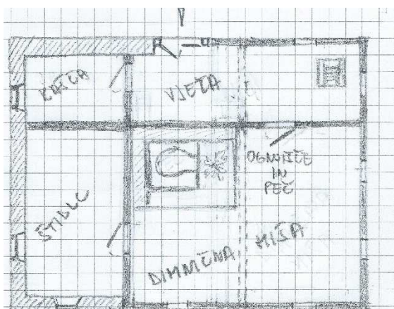
Slika 268: Tlorisa kleti in stanovanjskega nadstropja Pintarjave hiše v Križevi Dragi. Osnovne dimenzije objekta so 10,6 x 8,1 m.
