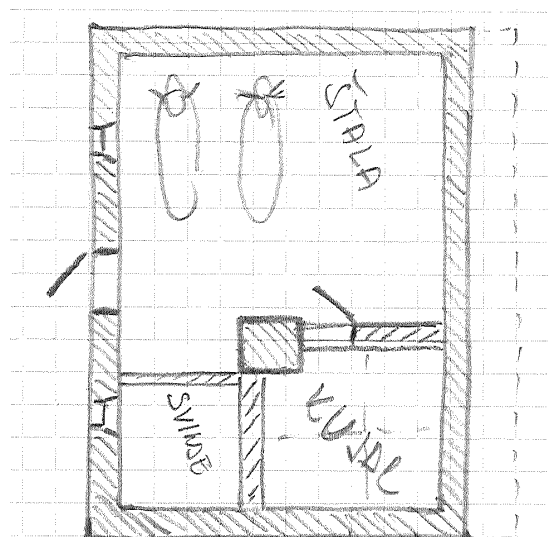
Slika 290: Tloris kleti Brenčkave hiše z Vrhov nad Trstjem. Zidovi so še stari, grajeni iz lokalnega kamna, le predelne stene so dozidane kasneje. Prvoten je tudi osrednji stebler. Dimenzije zidane kleti so približno 5,75x7,75m.
