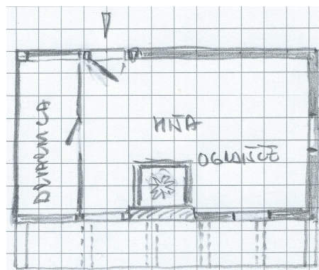
Slika 79: Rekonstrukcija tlorisa pritličja Ločičke hišice konec 19. stoletja, ko so stavbo povečali na sedanje dimenzije.
