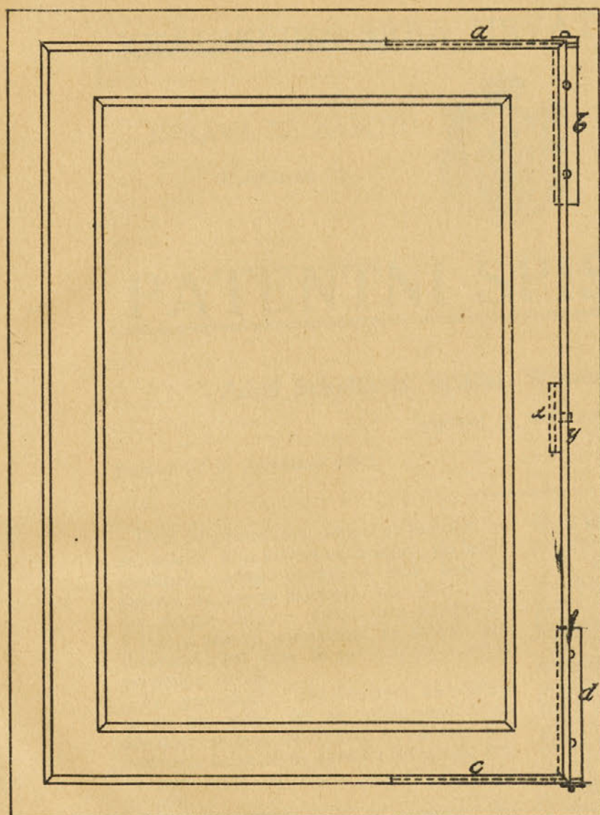
Pogled 1:3
