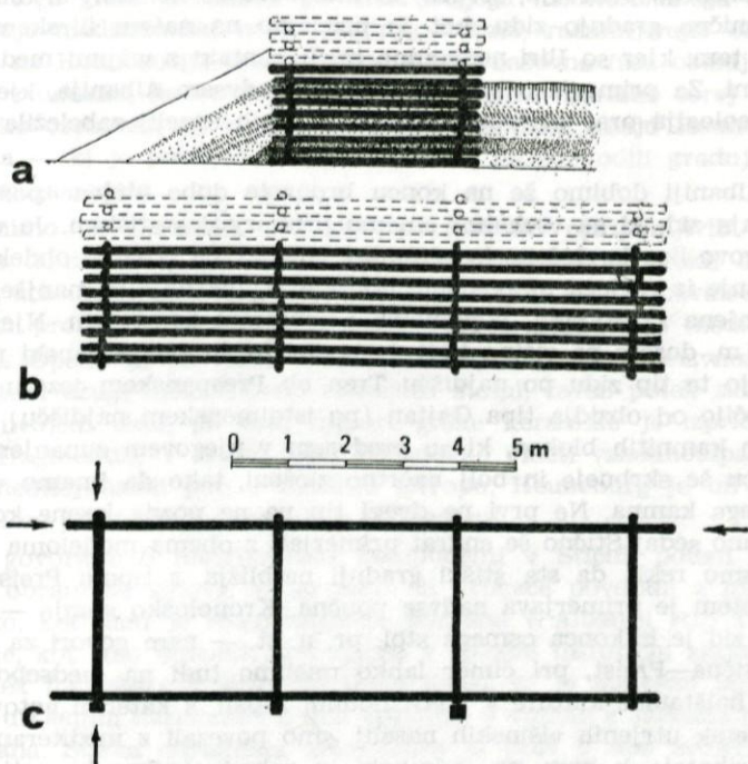
Sl. 2. Heuneburg. Sistem obzidja V. periode (tip Biskupin). Po Dehnu.
