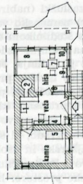
tloris nadstropja
