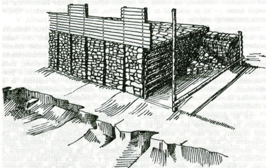
Sl. 3. Zid tipa Preist. Rekonstrukcija po ostankih v istoimenskem najdišču. Po Fischerju.
