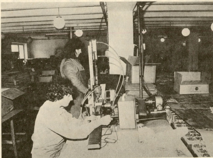
Z robljenjem plastičnih stročnic se zaključuje montaža baterij 2R 10
