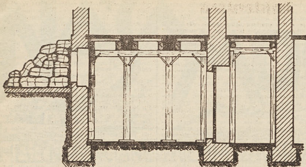
Zasilno ojačanje ravnega rebrastega železobetonskega kletnega stropa (V boljši izvršitvi, kjer je že tudi plošča zavarovana s plohi. Okno je izdelano s plohi in z vrečami peska)
