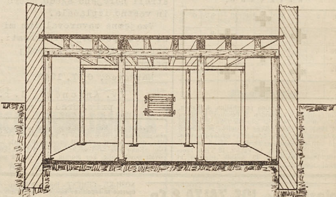
Preprosto podprtje ravnega rebrastega stropa v kleti
