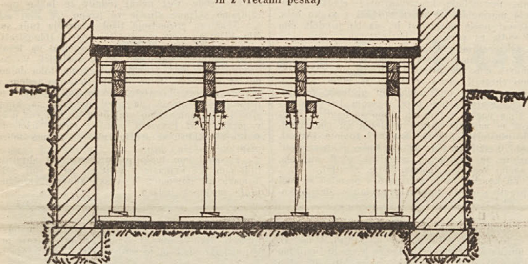
Zasilno ojačanje ravnega rebrastega železobetonskega kletnega stropa (V boljši izvršitvi, kjer je že tudi plošča zavarovana s plohi. Okno je izdelano s plohi in z vrečami peska)
