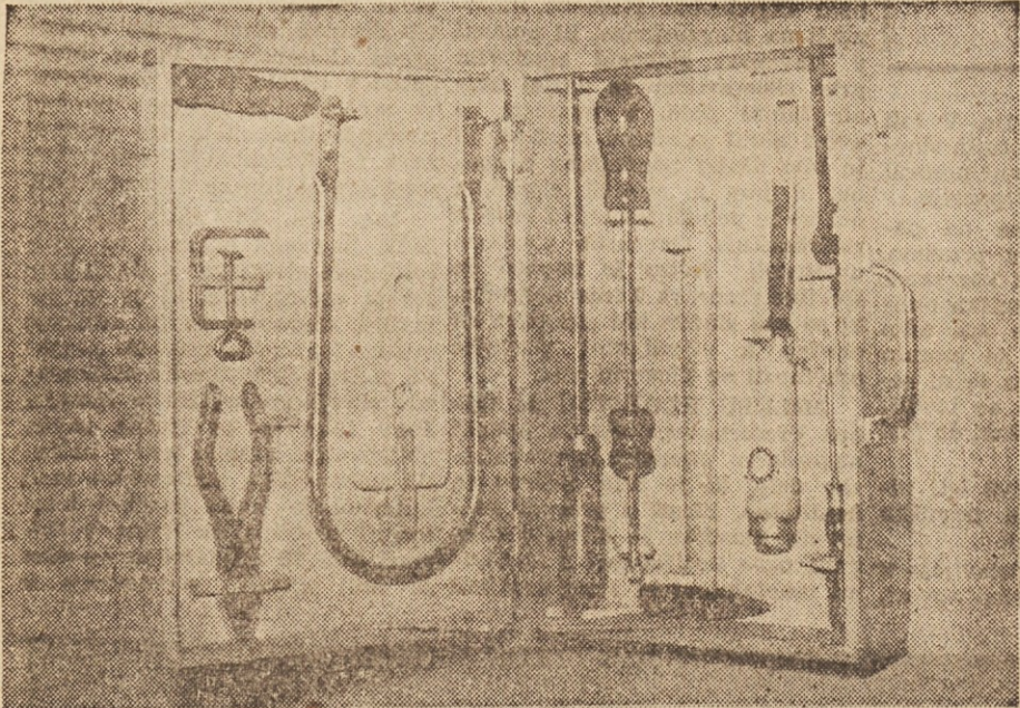
Garnitura orodja MT-104
