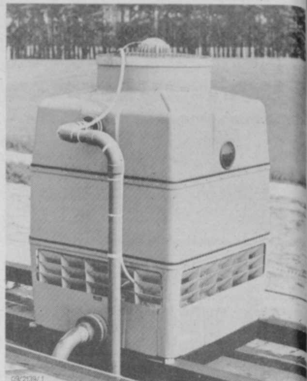
Hladilni stolp za povratno hlajenje vode z zmogljivostjo 121.300 kcal/h, izdelek TOZD ESOT, ki opravi tudi montažo in vso instalacijo od komandne plošče naprej.
