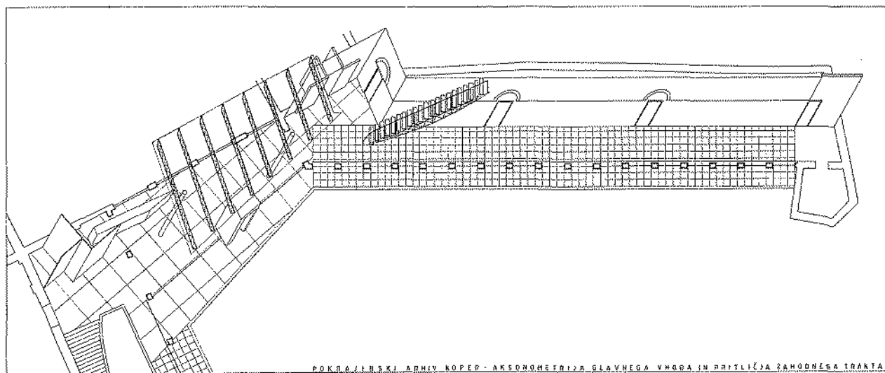
POKROBILNIŠKI ARHIV KOPER - AKSONOMETRIJA GLAVNEGA VHODA IN PRITLIČJA ZAHODNEGA TRAKTA
