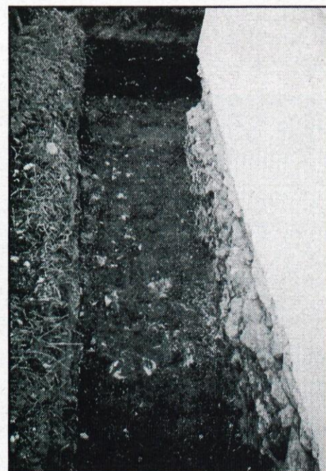
Na dnu jarka ob južni strani zidu je viden tloris starejše taze gradnje. foto: J. Škrlep
