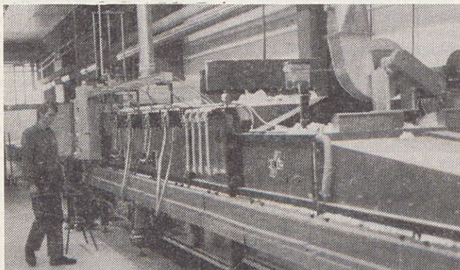
Sodobno linijo za ekskluzivno dekoriranje keramičnih ploščic zaključuje 10 metrov dolga enokanalna peč uglednega italijanskega proizvajalca Kemac, ki je ta hip najboljša tovrstna peč v svetu.
