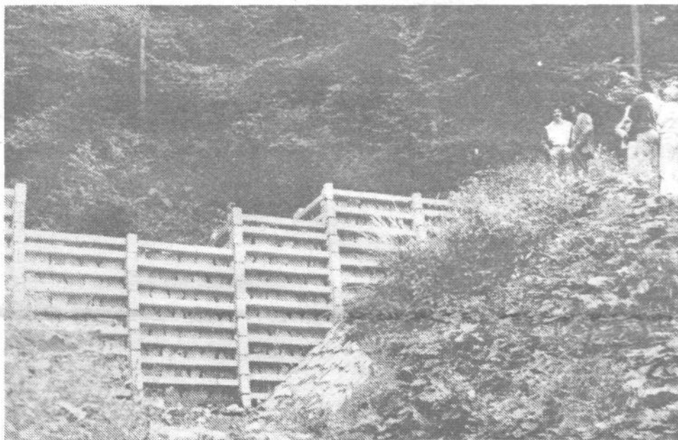
V Žirovnikovem grabnu so delavci Podjetja za urejanje hudournikov obnovili osem pregrad, ki so narejene iz betonskih kaš. Za tovrstni objekt uporabljajo slovenski izraz »kašta« po celem svetu.
