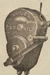
Br. 112d: Klaniška dizalica sa automatskom kočnicom, nosivost kg 1000, cijena Din 5500.
