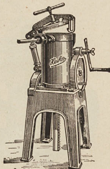
Br. 194a: Stroj za punjenje kobasica, sadrž. oko 15 20 25 30 lit. Cijena Din 8500 9600 11.000 12.800
