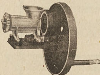
Br. 212a: Mesorezni stroj za ručni ili motorski pogon sa zupčastim točkovima, br. 32 Din 1200, br. 42 Din 2000.
