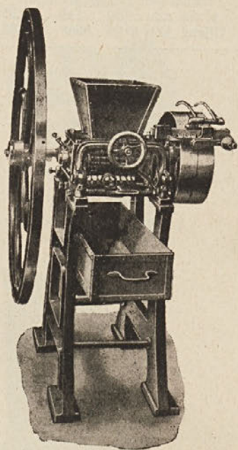
Br. 195a: Gnječilica na motorski pogon sa 9 11 15 noža Cijena Din 7800 9400 11.800 sa 19 23 31 noža Cijena Din 16.000 19.000 27.000
