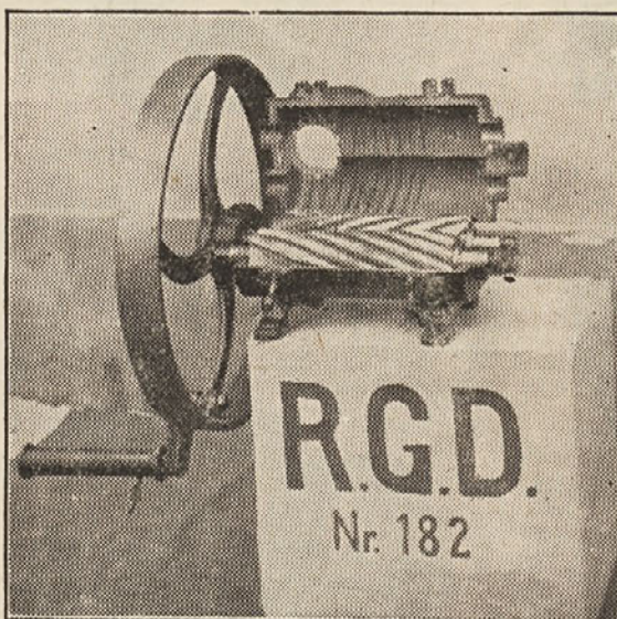
Br. 182: Gnječilica sa točkom na ručni i mehanični pogon ujedno, cijena Din 2400.
