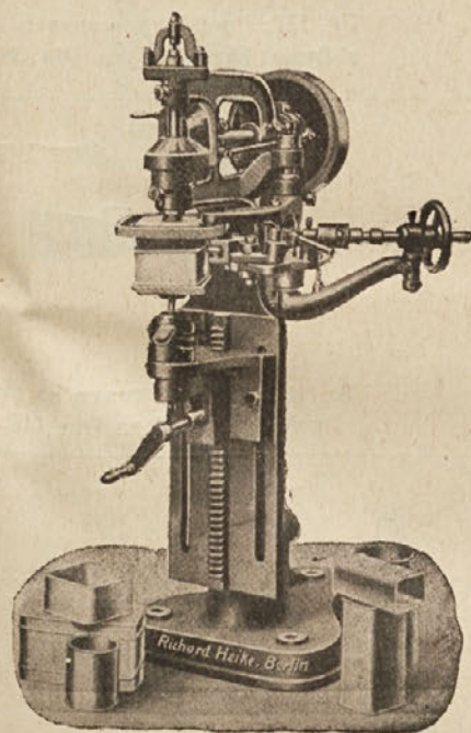
Br. 351: Kombinirana univerzalna mašina za zatvaranje raznih konzerva. Cijene na upit.
