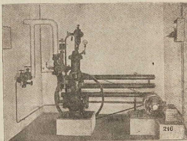
Br. 216: Stojeći kompresor za veće hladionice ili tvornice leda. Cij. prema kalkulaciji.
