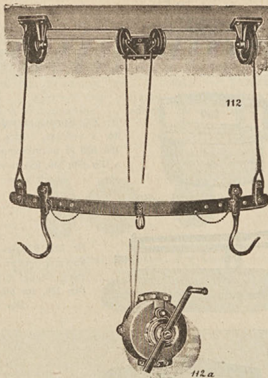
Br. 112 i 112a: Klaniška dizalica, cijena za izradbu prema slici Din 7500, za nosivost 1000 kilograma.
