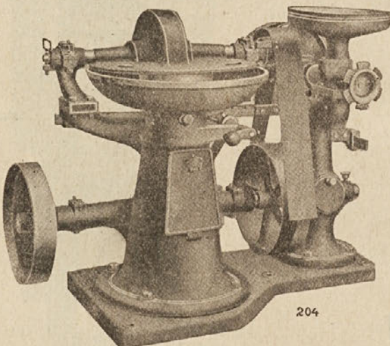
Br. 204: Blitz i Wolf ujedno sa montiranim motorom ili bez motora za transmijski pogon. Cijene na upit.
