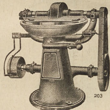
Br. 203: Stariji model Blitz; cijene i veličine kao kod modela »Căsar« pod br. 203a.
