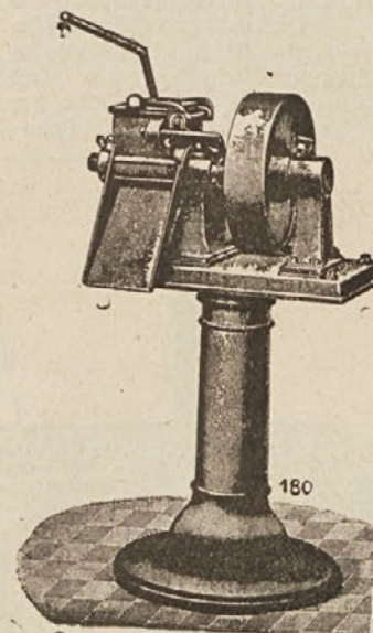
Br. 180: Mlin za kosti, 2 veličine, cijena Din 4800 i 6800. Može se dobiti i na stalku sa četiri noge.
