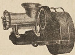
Br. 212c: Stroj br. 32 na motorski pogon, cijena Din 1400, br. 42 Din 2200.
