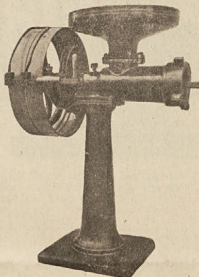
Br. 209: Wolf za velike radnje na motorski pogon sa zaštićenim pužem (najnoviji puž!), promjer ploča 130 mm, cijena Din 6800.
