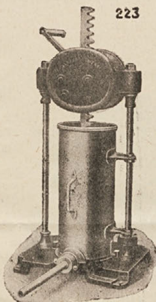
Br. 223: Stroj za punjenje kobasica. Sadržina litara 6 9 12 16 Cijena Din 1500 2000 2400 2600.
