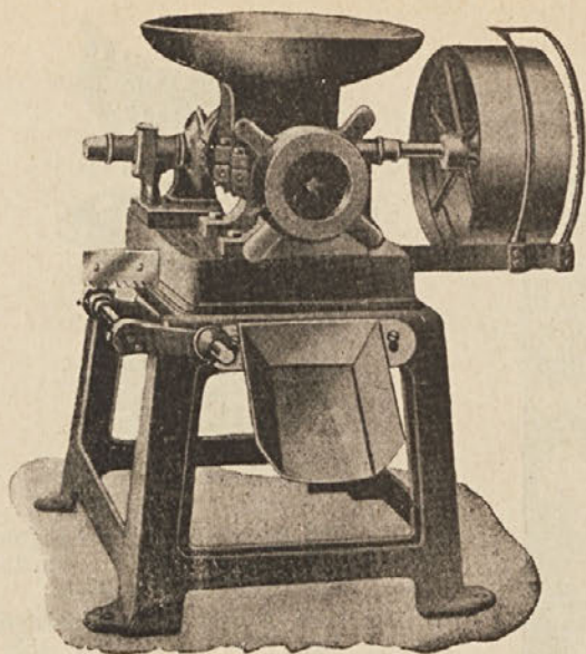
Br. 336: Veliki Wolf starije konstrukcije, veličina mm 125 150 200 Cijena Din 8500 19.000 26.000.
