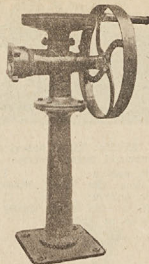
Br. 208: Wolf sa stalkom i točkom na ručni i mehanični pogon, najmodernija konstrukcija, promjer ploča 98 mm, cijena Din 2600. Isti Wolf sa 2 točka (puni i prazni tek) Din 3800.
