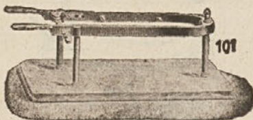
Br. 101: Kliješta za šunku, poniklovana, dužina 14 coli, bez držaka; cijene: na ploči od drveta Din 220, na ploči od mermera Din 260.
