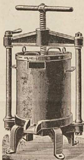
Br. 193a: Presa za čvarke, osobito jake konstrukcije, sadržina 15 25 45 lit. Cijena Din 2000 3000 4000.
