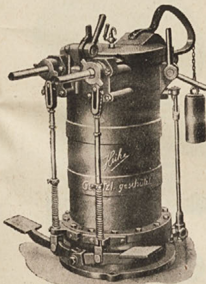
Br. 194b: Stroj za punjenje kobasica, sadržina 75 litara, cijena Din 25.000.
