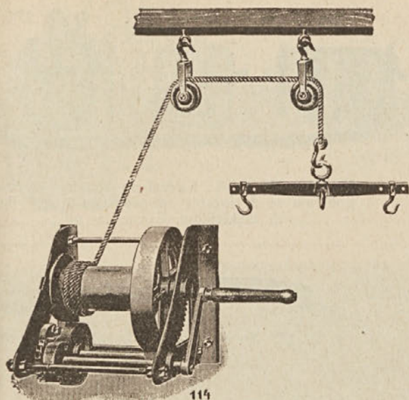
Br. 114: Jednostavna klaniška dizalica, nosivost kg 1000, cijena ukupno Din 4000.
