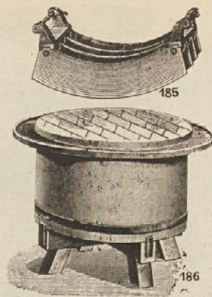
Br. 185: Njhaći noževi za ručni pogon, 3 4 5 6 noža. Cijena Din 2400 2800 3200 3800 Br. 186: Panj za ručne njhaće noževe. promjer mm 1000 1150 1400 1550 Cijena Din 3200 3800 4200 4600.
