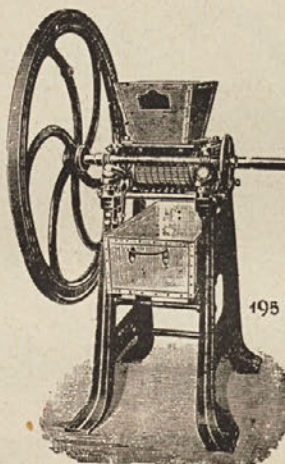
Br. 195: Gnječilica na ručni pogon sa 9 11 15 noža Cijena Din 7600 9200 11.600
