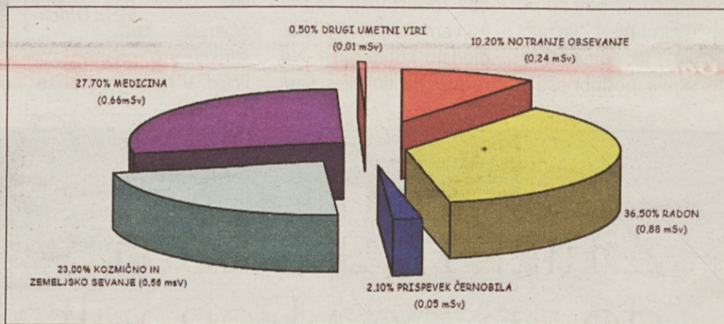
Obsevanost prebivalstva v Sloveniji, skupaj 2,4 mSv (milisieverta) na leto (Delo z viri sevanj, 2006)
