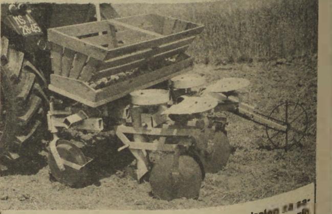
Sadilnik TS-2-SCT je traktorski priključek prirejen za sajenje krompirja, okopavanje krompirja, koruze in drugih poljščin. Je prirejen za dvovrstno sajenje, kot kultivator in osipalnik pa za trivrstno okopavanje oziroma osipavanje. Stroj priključimo na traktor s standardnim orisnim kategorije I. in II. Potrebna pogonska moč je 15 KS oz. 11 kW.
