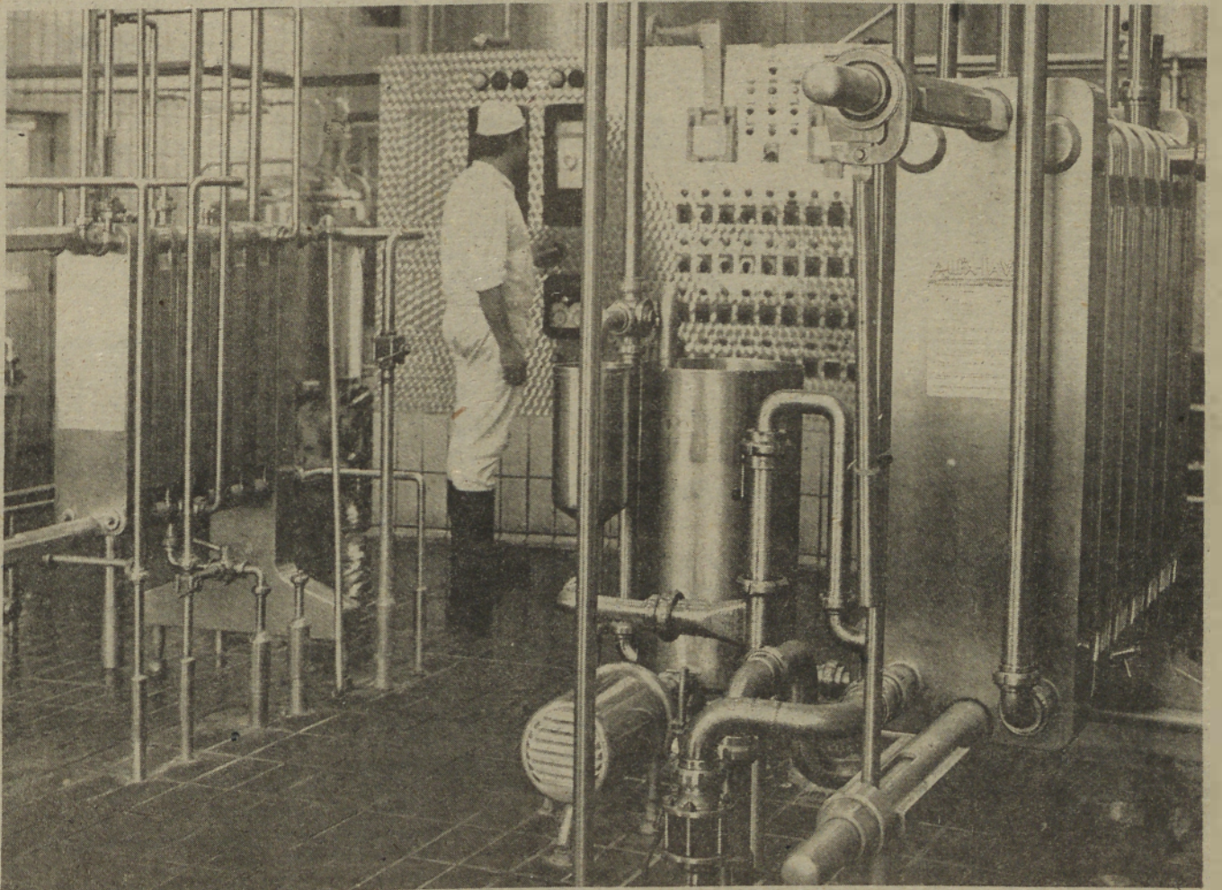
Naprave za predelavo mleka v tovarni mlečnega prahu v Murški Soboti.
