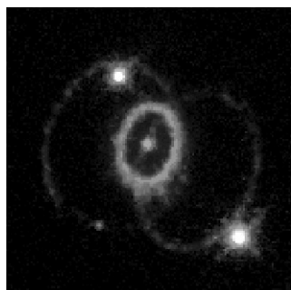
Ostanki Supernove iz leta 1987
