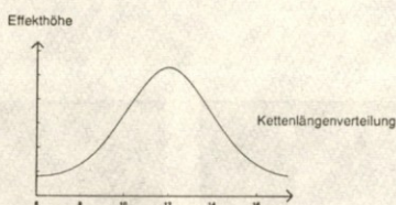
Slika 3 Perfluoralkylmercaptane und Alkohole
