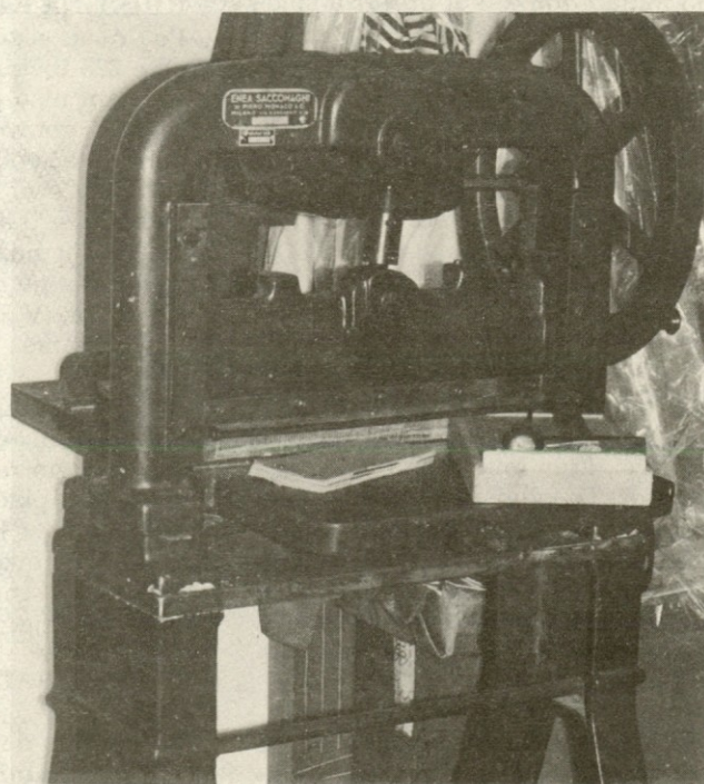
Stroj za izdelavo vzorcev v vzorčnem oddelku je star okrog 27. let in popolnoma nemehaniziran. Vzorce je treba rezati z ročnim pogonom stroja. Uporabljajo se še pripomočki kot kladivo, deska in pribijač.
