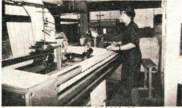
Avtomat za robljenje po dolžini v šivalnici frotirja
