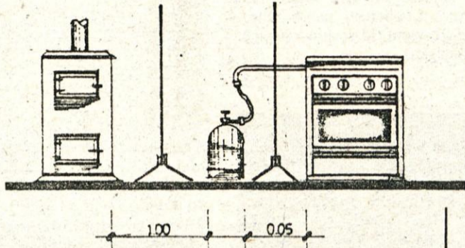
Postavitev plinske jeklenke
