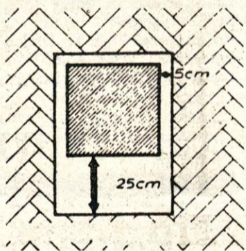
Velikost zaščite gorljivih tal
