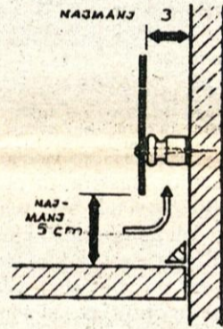
Oddaljenost zaslona od gorljive stene
