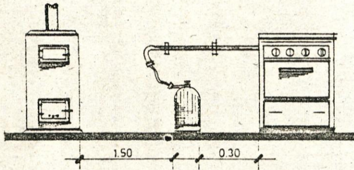
Postavitev plinske jeklenke
