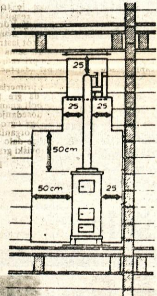
Varnostne razdalje od gorljivih sten z zaslonom ali brez njega
