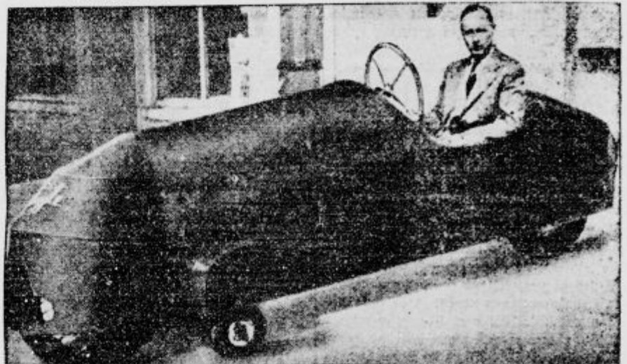
Avto na dve kolesa je zgradil ameriški tovarnar Grady Tuigle. Majhna kolesca ob strani drže avto v ravnotežju samo, kadar stoji. Med vožnjo se dajo stranska kolesa potegniti v trup avtomobila.
