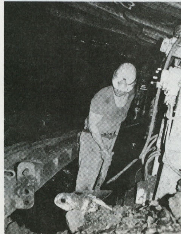
Dandanes v velenjskih jamah ni več redkost odkopna mehanizacija
