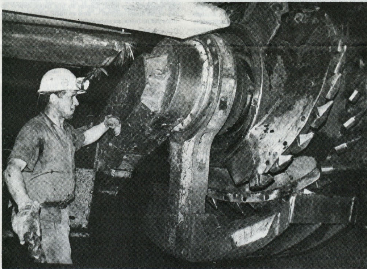
Današnje dni je na fronti naših odkopov že marsikje najprej stroj
