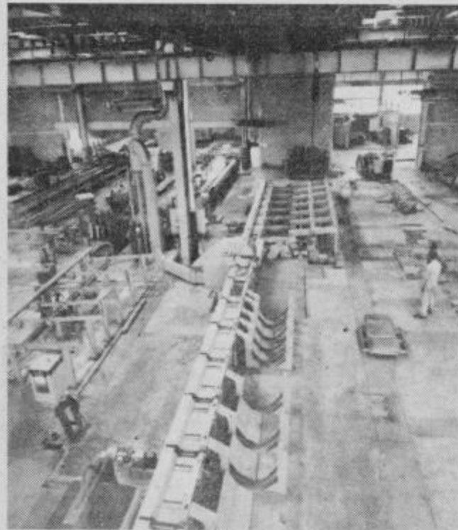
Novi jeklovlek v štorski železarni: proizvodne prostore so zgradili v manj kot dveh letih in tudi že montirali večino starih in novih strojev.
