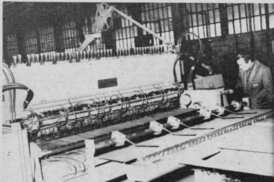
Najmodernejši varilni stroj Žične Celje s katerim varijo armaturne mreže za gradbeništvo
