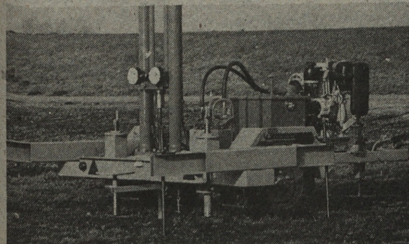
Statičen penetrometer z maksimalno silo 200 kN poriva v zemljo jeklene palice, dolžine 1 m
