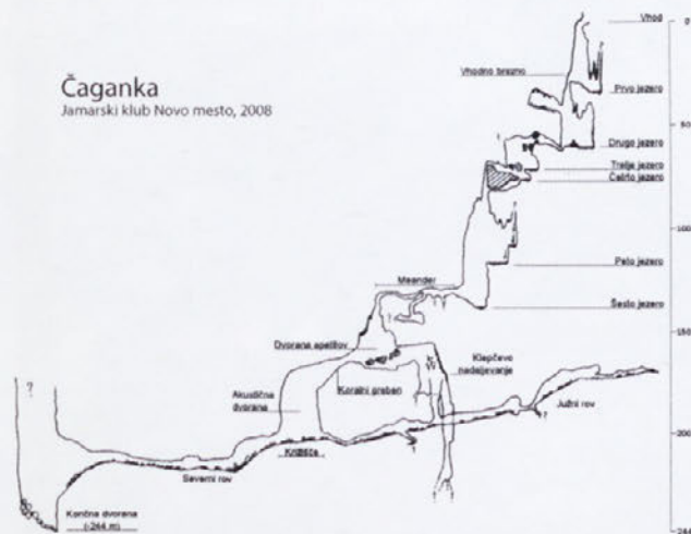
Iztegnjeni profil jame. Risala Borivoj Ladišič in Srečko Vidic.
