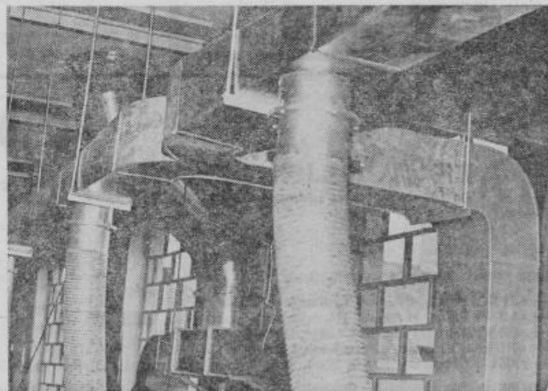
Odsesovanje od brusilnih strojev
