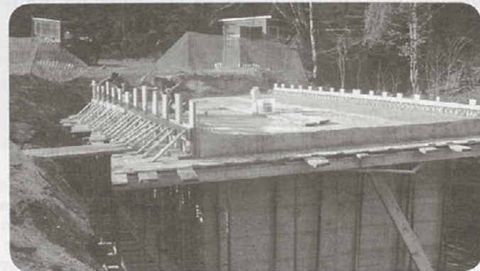
Gradnja novega mostu preko reke Jevniščice
