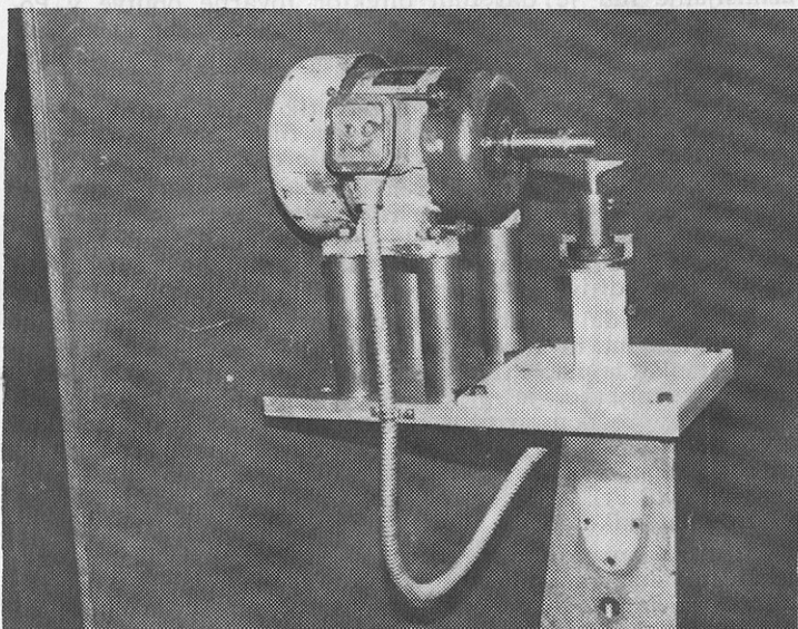
Izum Antona Zupana. Stroj za izrez kopic in podloge pri novofleks obutvi.
