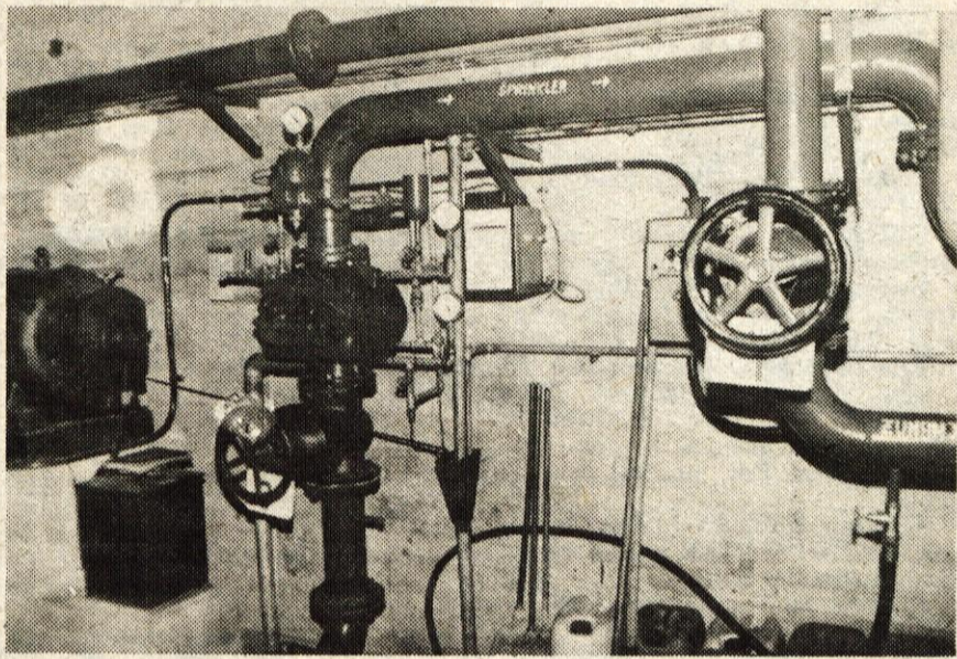
Strojica bazena sprinkler sistema za gašenje.
