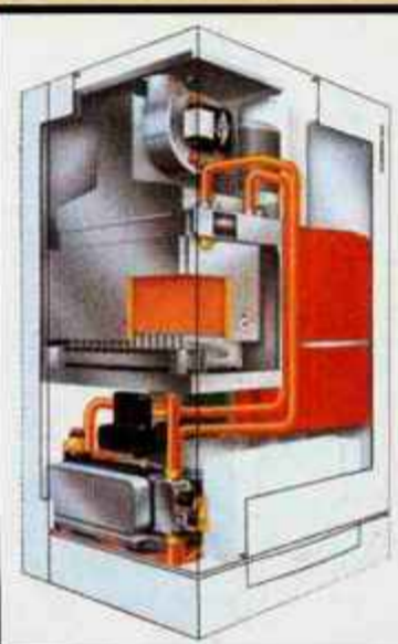
VITOPEND 222 10,5 do 24 kW (30 kW-booster obratovanje za sanitarno vodo)
