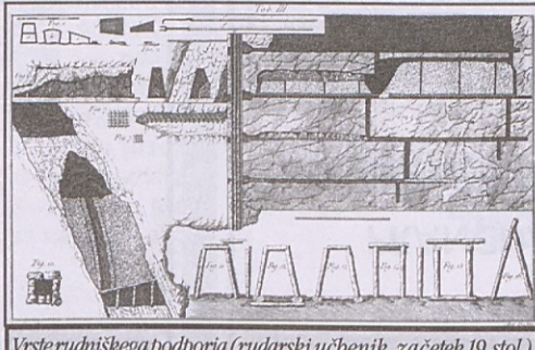
Vrste rudniškega podpora (rudarski učbenik, začetek 19. stol.)
