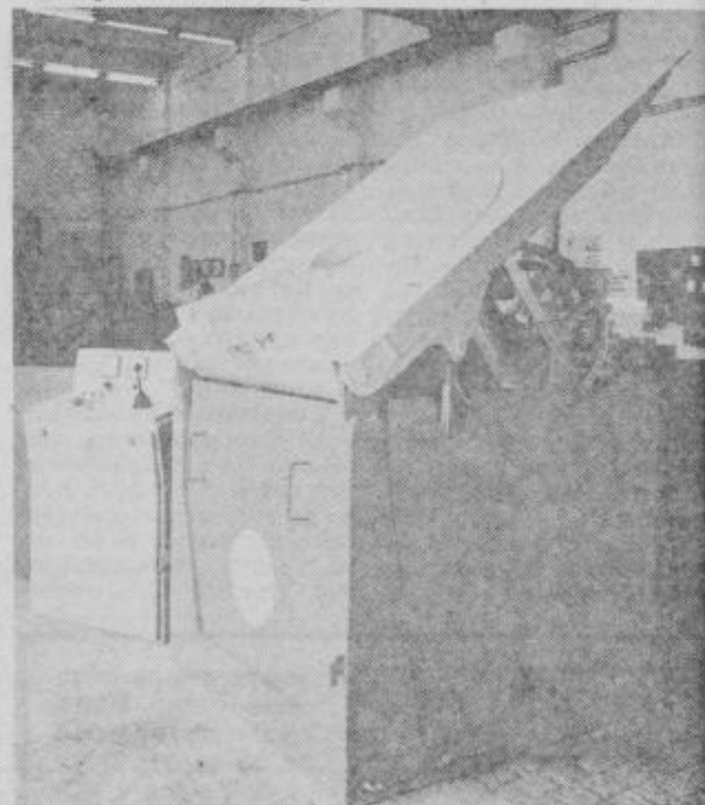
Indukcijska lončna peč 250 kg.
