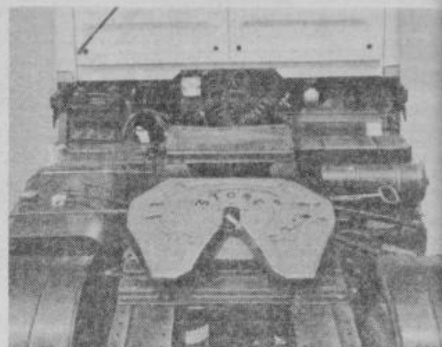
Priklopno sedlo vlečnega vozila.
