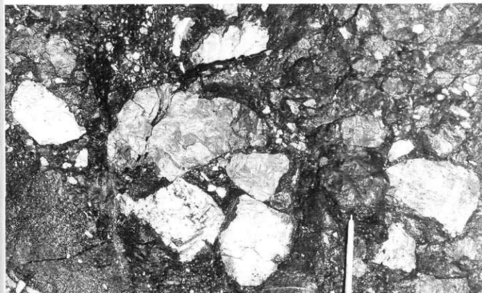
Dolomitna blokovna breča z bituminozno-muljasto osnovo. Neobičajna kamnina zapolnjuje najgloblje dele idrijskega srednjetroasnega tektonskega jarka, v katerem je nastalo idrijsko rudišče.
