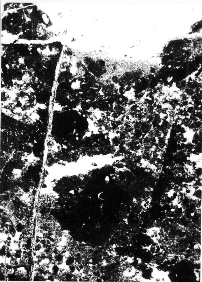
Geopetalna tekstura – izsušitvena pora z notranjim sedimentom (razlaga v tekstu). V zgornjem desnem delu je viden del izsušitvene pore (belo). Dno pore pokriva drobnozrnat karbonat – dolomikrit (sivo zrnato polje) v obliki internega sedimenta. Mikroskopska fotografija dela zbruska (opis v tekstu) dolomitne kamnine. Daljši rob slike = 5,5 mm.
