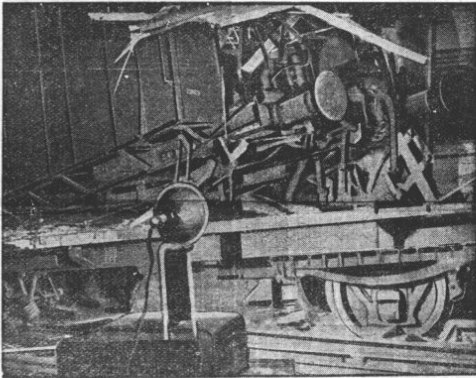
Pri Perpignanu v južnih Pirenejih se je zaradi izpodkopenega železniškega nastpa iztril vlak in lokomotiva se je zarila globoko v blato.
