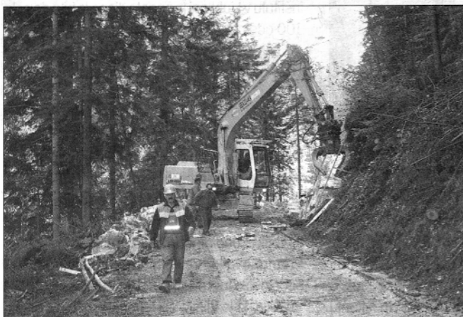
Gradnja podpornih zidov na cesti ob Rogačniku (foto: Marija Lebar)
