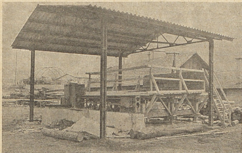
Na prostoru lesnega skladišča v Trbovljah je v teku gradnja cirkularja za vzdolžno paranje jamskega lesa za potrebe mehaniziranih odkopov v jamah.
